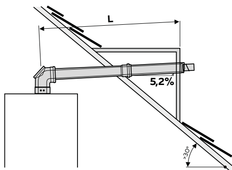
Instalações C13x DN 60/100 e 80/125
