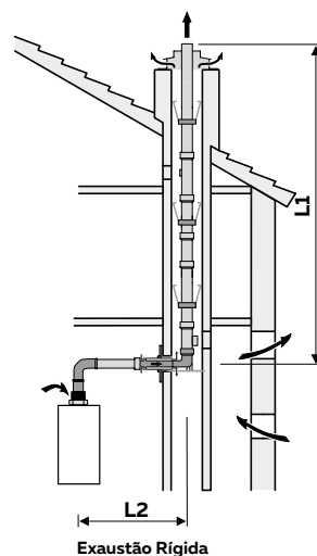
Instalações B53x DN 60 e DN 80
