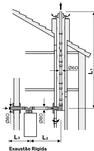
Instalações C53x DN 60 (admissão DN80)
