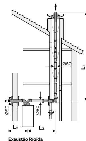
Instalações B53x DN 60 e DN 80
