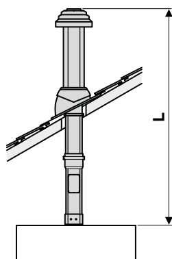
Instalações C33x DN 60/100 e 80/125
